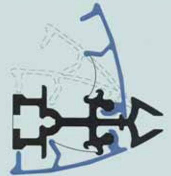
Profil Klapprahmen
